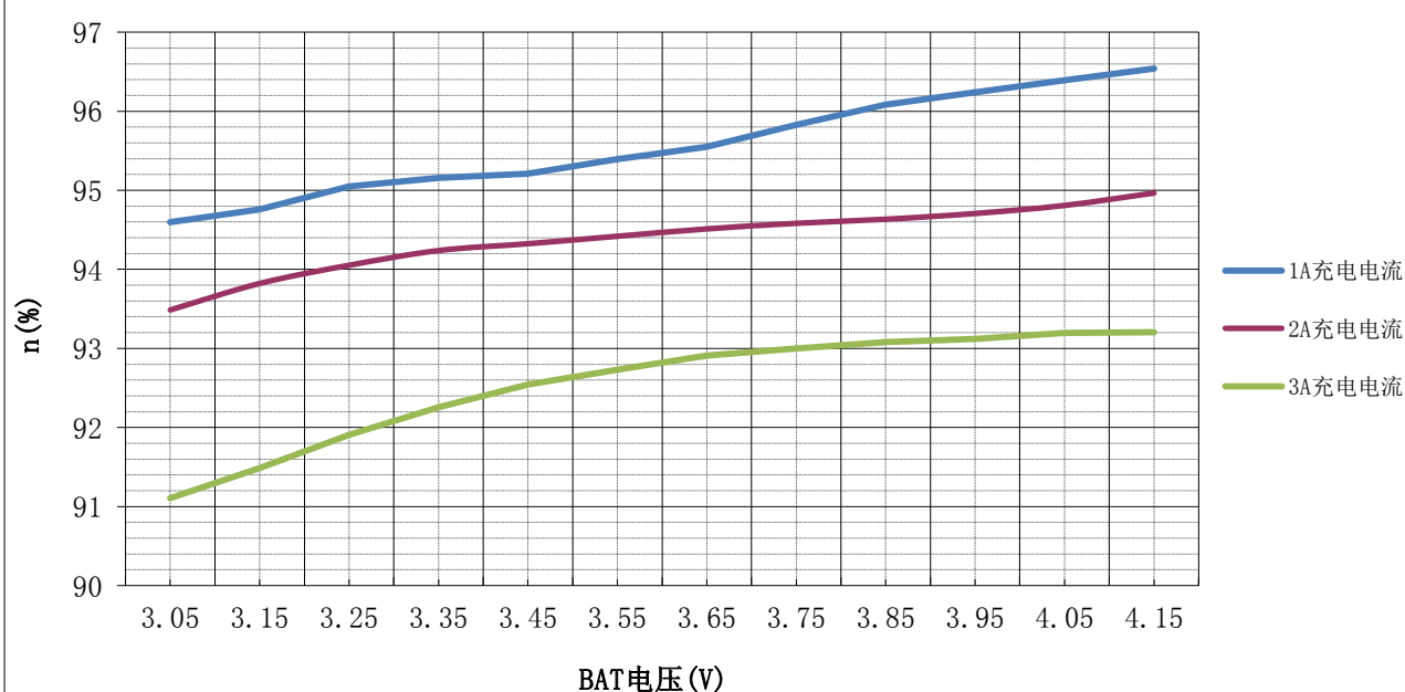
IP2312充电效率曲线 VIN=5V
